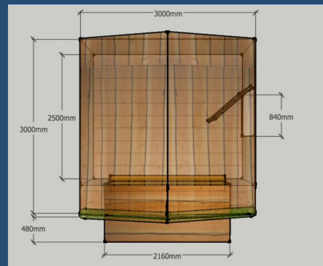
Grondplan chalet:
